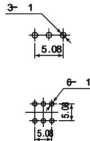
取付穴参考寸法 Mounting Hole
